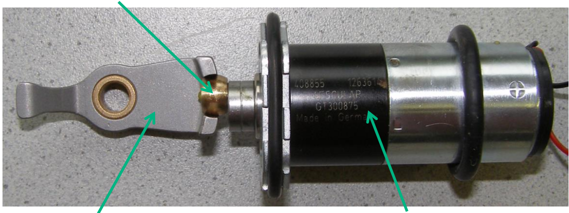
GT300880 LEVIER POUR CALOTTE
